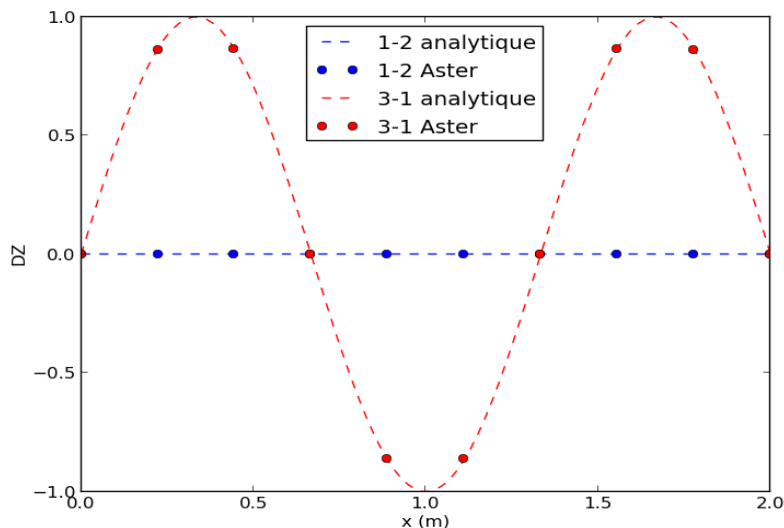
Figure 3.2-1 - Déformées modales suivant le grand axe médian.
