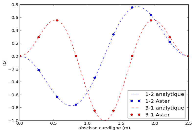
Figure 10.2-3 - Déformées modales suivant la diagonale.
