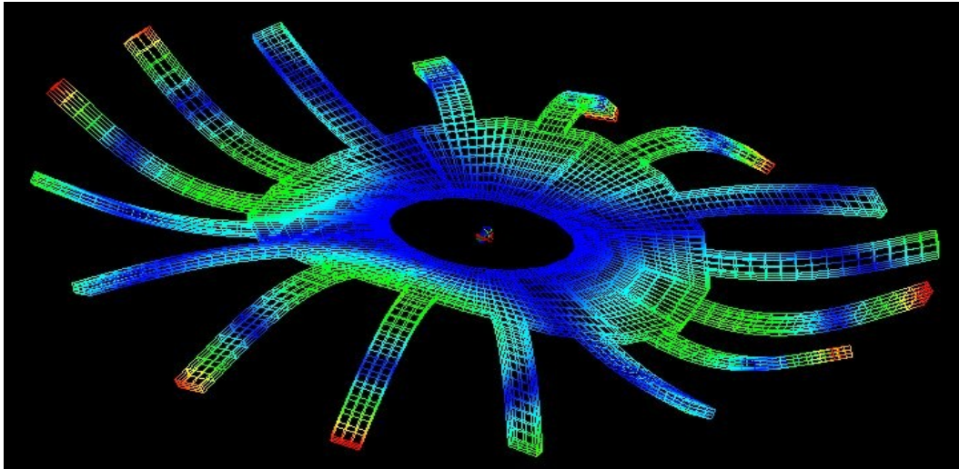
Mode 5 : 80.2363 Hz
