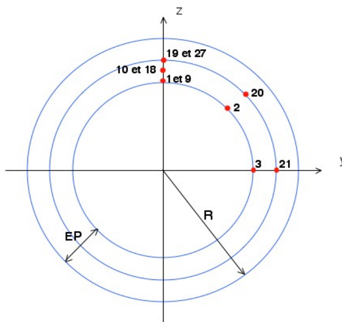
Figure : Discrétisation de la section, position de quelques sous-points
