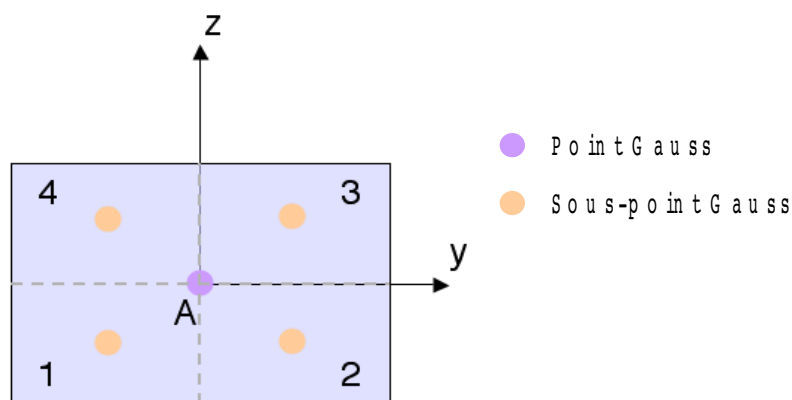
Figure 2.2-a : position des sous-point dans la section
