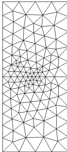
Figure 3.2-a: Maillage pour le problème 1
