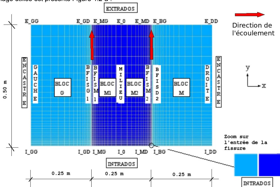
Figure 4.2-a : Maillage complet
