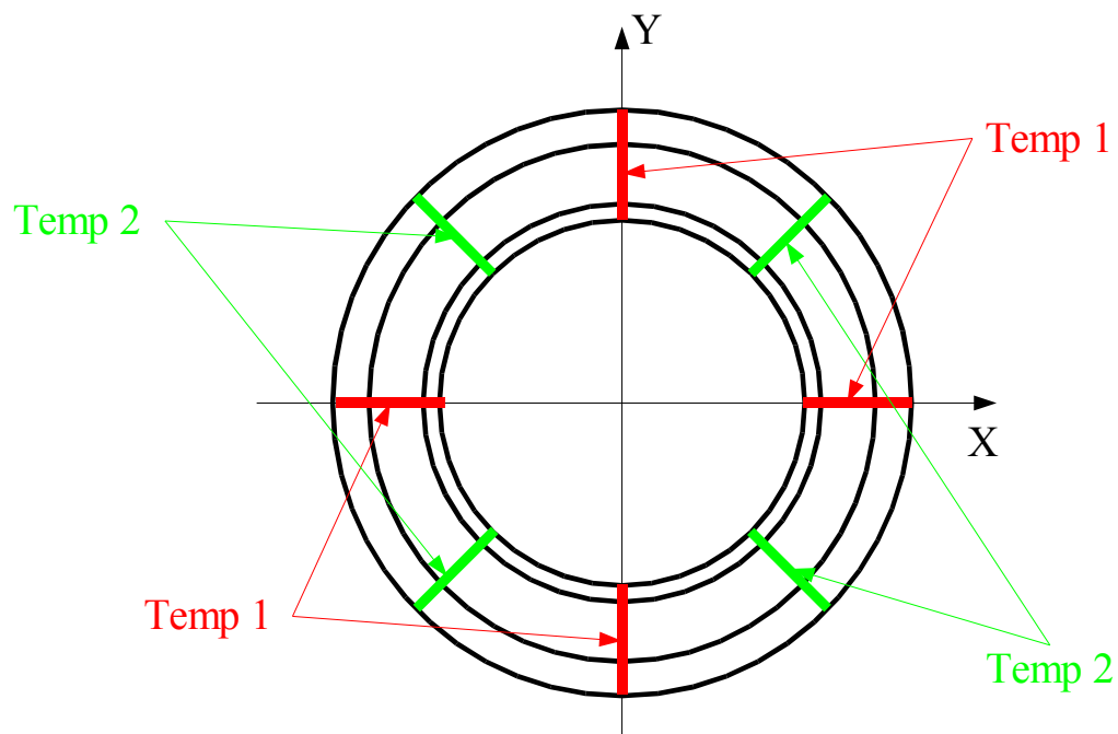
Figure 1.3-a : Vue de dessus, avec les conditions en température imposée.
