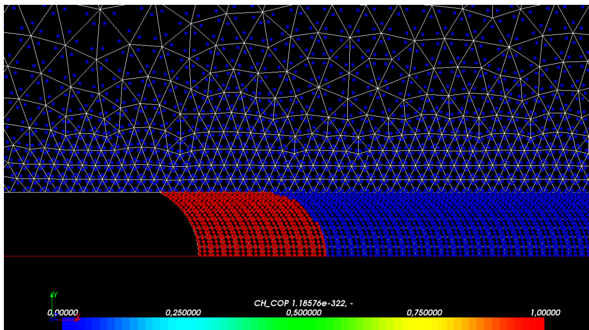
Figure 4-2 - Champ de visualisation des copeaux.
