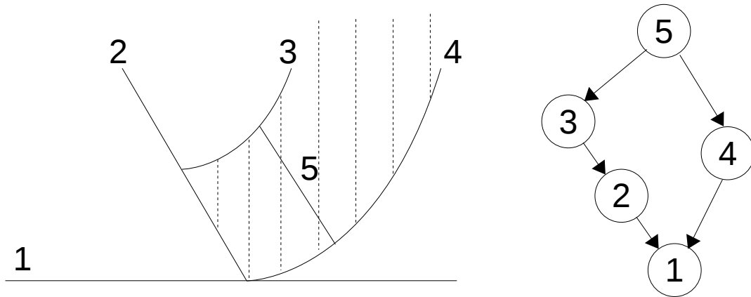
Figure 3.8-2 : Réseau de fissures à gauche, arbre de hiérarchie à droite indiquant qui se branche et permettant d'établir les relations d'ordre pour les définitions de fissure et l'utilisation de l'opérateur JONCTION.
