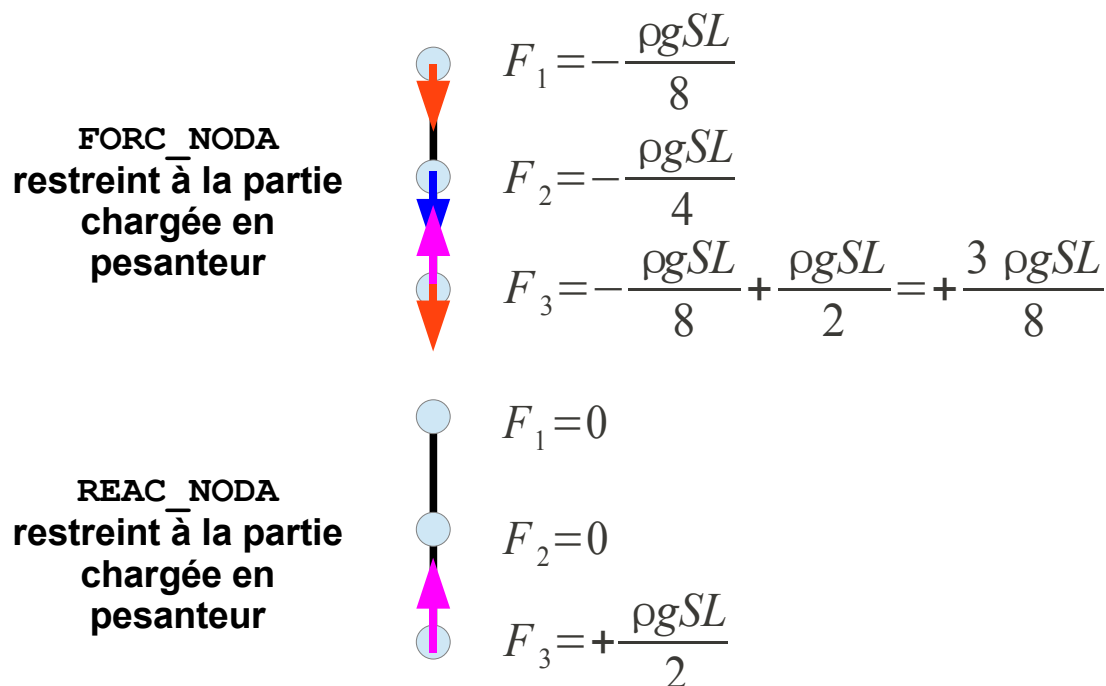
Figure 2.9.4-2: isolation d'une partie de la structure
