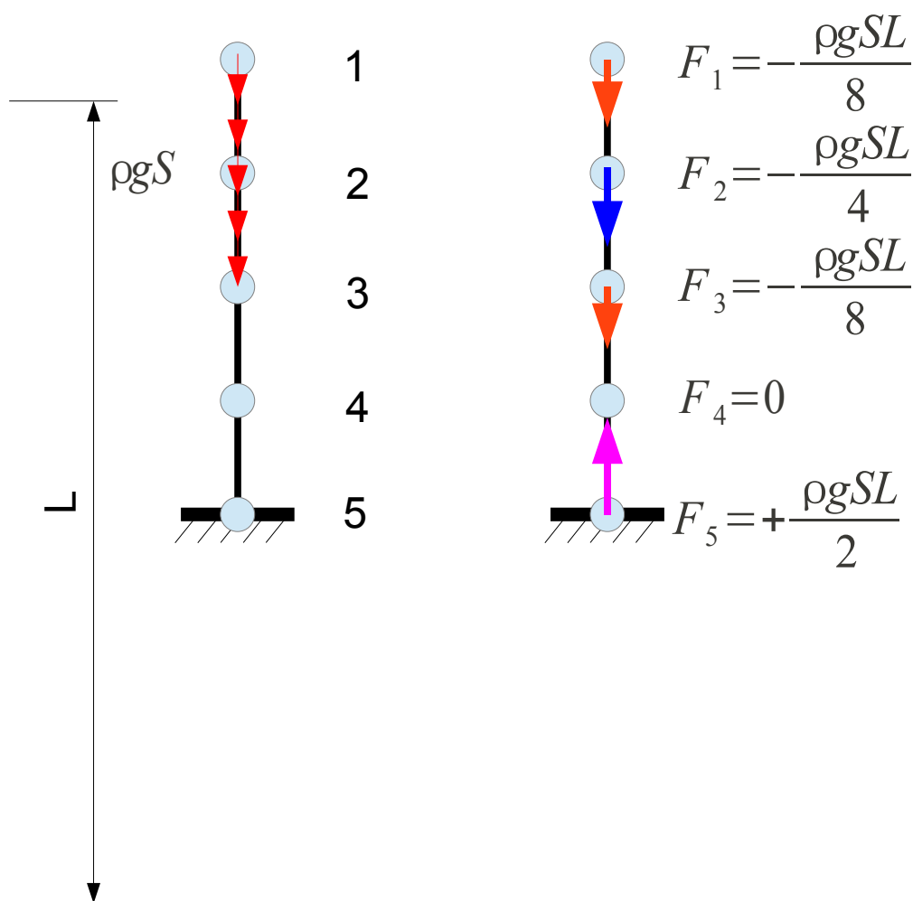
Figure 2.9.4-1: structure sous chargement réparti (gauche), FORC_NODA (droite)
