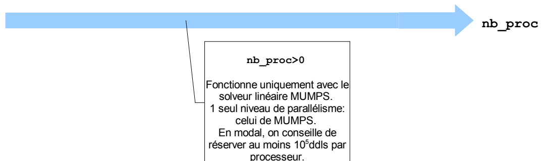
Figure 3.8-3. Périmètre d'utilisation avec NIVEAU_PARALLELISME='PARTIEL'.
