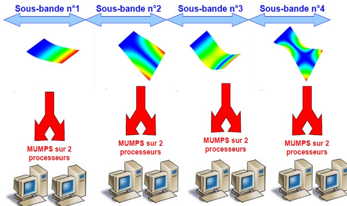
Figure 3.8-1. Exemple de distribution des calculs de MACRO_MODE_MECA sur 8 processeurs avec un découpage en 4 sous-bandes fréquentielles.
