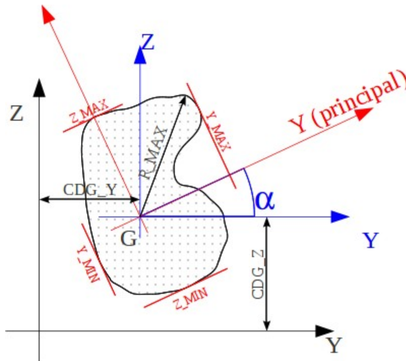
Figure : Définition des grandeurs géométriques relatives à une section de poutre.
