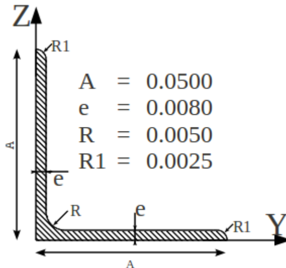
Figure : Cornière à ailes égales 50x50x8.
