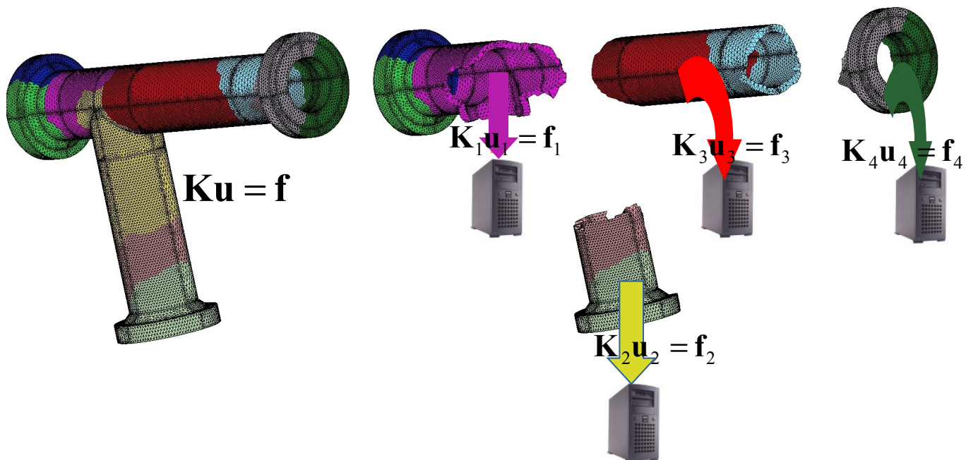
Figure 7.3-1: Principe de la décomposition de domaines de type FETI illustré sur une zone de mélange d'un circuit RRA.
