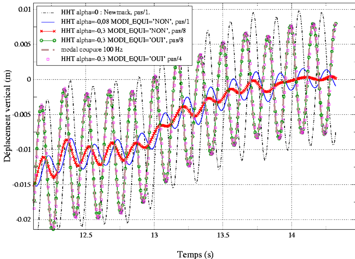
Figure 3.3.2-c : comparaison globale du comportement des schémas en temps.
