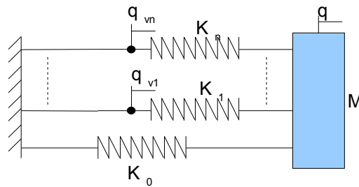
Figure 3: Calcul des modes « encastres ». Représentation du système à un seul degré de liberté équivalent.
