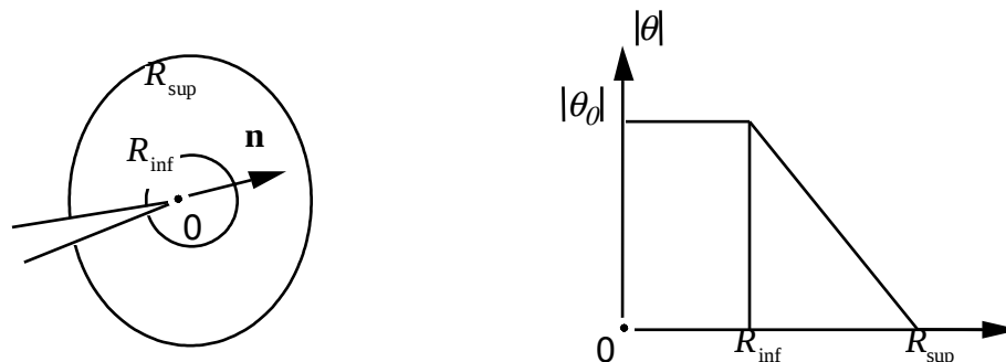
Figure 4.1.2-1: Définition géométrique du champ \theta
