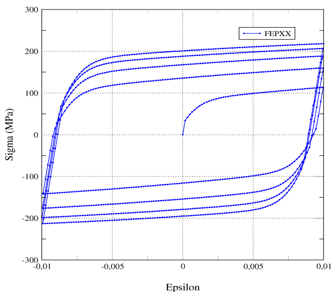
Essai cyclique DEPS=+/-1%
