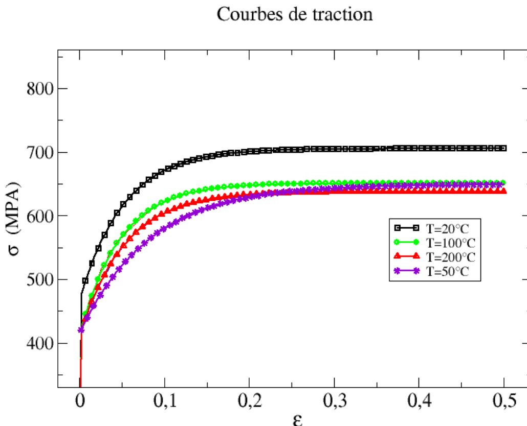
Figure 4.2-a . Courbes de traction en fonction de la température – résultat à 50^\circ
