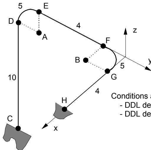
Modélisation TUYAU (SEG3)
