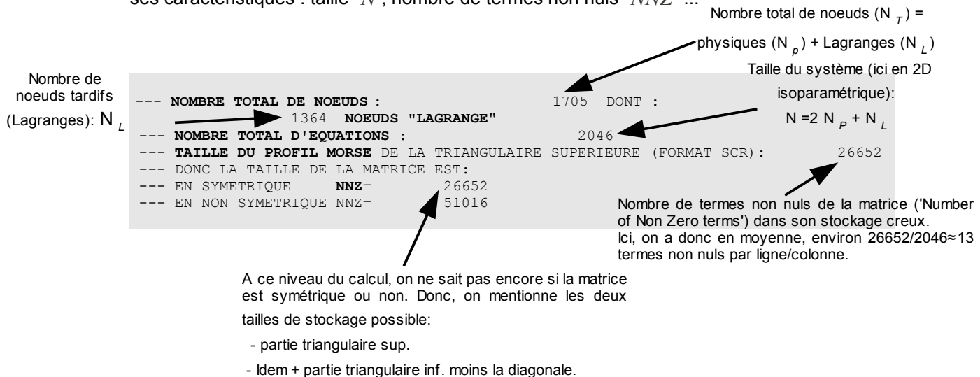
Figure 3-a : Caractéristiques du système linéaire en cours d'assemblage dans une commande Aster type STAT_NON_LINE ou THER_LINEAIRE (extrait du .mess ).
