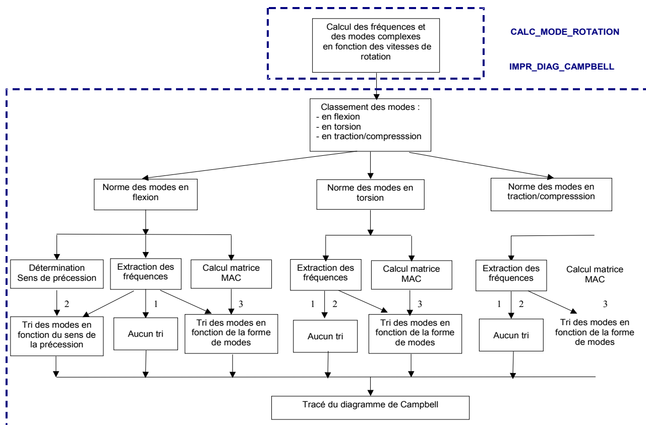
Figure 2-a-a : Organigramme du diagramme de Campbell
