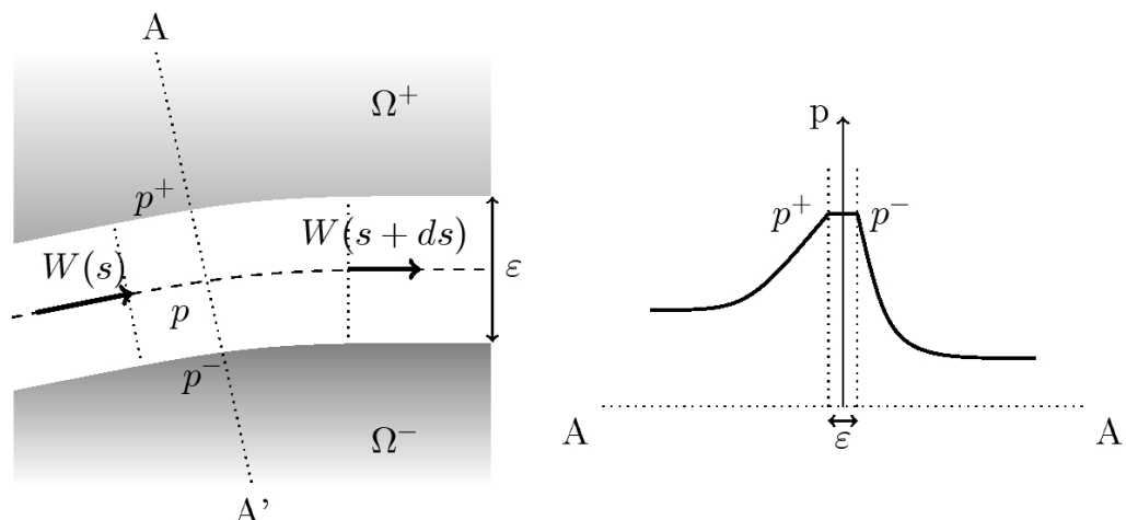
Illustration 3.2.1: conservation de la masse dans la fissure (à gauche) et profil typique de pression à travers l'interface (à droite)
