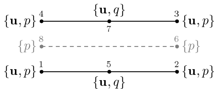
Illustration 5.2.1: Vue "éclatée" de l'élément de joint avec couplage hydro-mécanique et sans propagation
