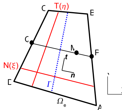
Figure 6: Paramétrage de l'élément à discontinuité
