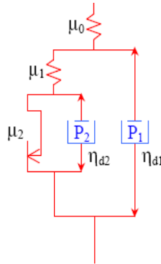
Figure 2.5.1.2-a : Représentation viscoélastoplastique déviatorique (VEP d )
