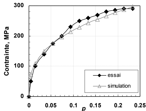
Figure 2-b : Loi d'écrouissage de l'acier non corrodé
