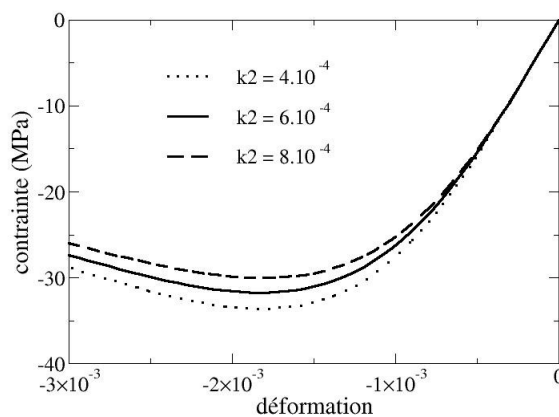
Figure 4.3.2.2-c : Dépendance de la réponse en compression simple vis-à-vis de k_2 ( E = 32000 MPa, \nu = 0.2 , k_0 = 3.10^{-4} MPa, k_1 = 10.5 MPa, \gamma_d = 6.10^{-2} MJ/m 3 )
