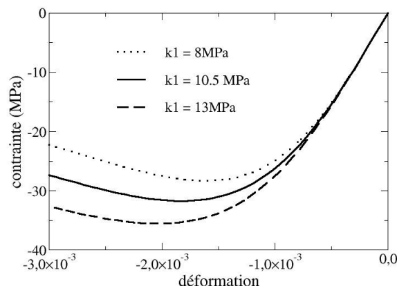
Figure 4.3.2.1-a : Dépendance de la réponse en compression simple vis-à-vis de k_1 ( E = 32000 \text{ MPa} , \nu = 0.2 , k_0 = 3.10^{-4} \text{ MPa} , k_2 = 6.10^{-4} , \gamma_d = 6.10^{-2} \text{ MJ/m}^3 )
