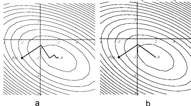
Figure 3.1-2. Convergences comparées, sur l'exemple n°1, de la Steepest Descent (a) et du GC (b).
