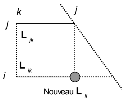
Figure 4.2-1. Phénomène de remplissage lors de la factorisation.
