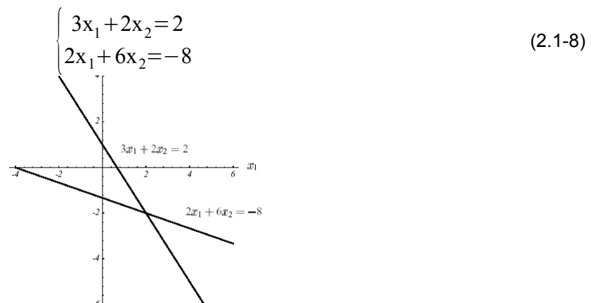
Figure 2.1-2. Résolution de l'exemple n°1 par intersection de droites.
