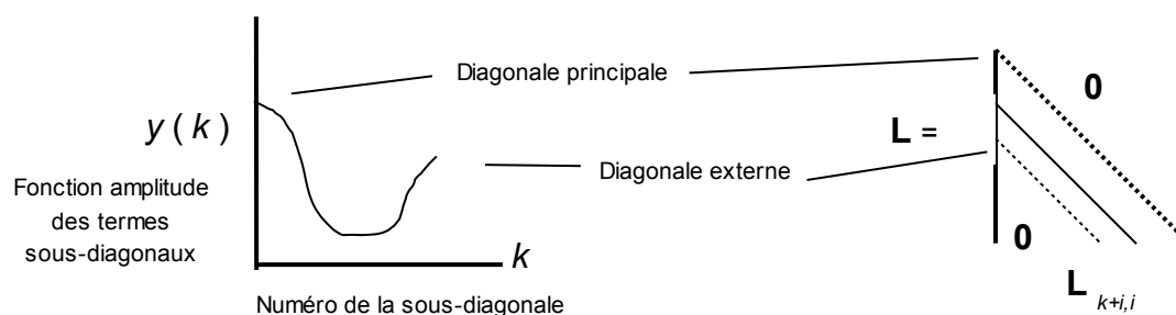
Figure 4.2-3. Importance relative des diagonales de L
