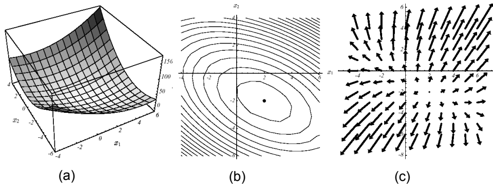
Figure 2.1-1 . Exemple de J quadratique en N=2 dimensions avec \mathbf{K} := \begin{bmatrix} 3 & 2 \\ 2 & 6 \end{bmatrix} et \mathbf{f} := \begin{bmatrix} 2 \\ -8 \end{bmatrix} : graphe (a), lignes de niveaux (b) et vecteurs gradient (c). Le spectre de l'opérateur est (\lambda_1; \mathbf{v}_1) = (7; [1, 2]^T) et (\lambda_2; \mathbf{v}_2) = (2; [-2, 1]^T) .
