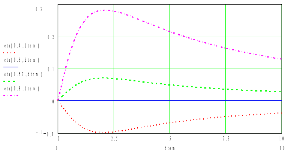
Figure 6.2-b : Coefficient d'amortissement numérique \eta en fonction de \omega \cdot \Delta t \in [0.0, 0.4] , pour \theta = 0.40, 0.50, 0.57, 0.80 .
