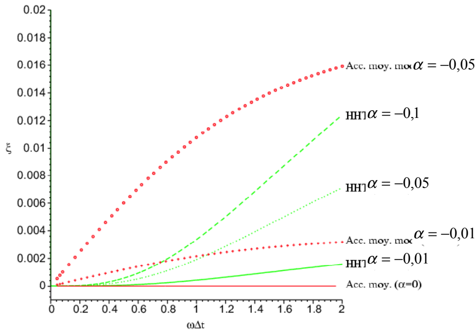
Figure 5.4-a : Taux d'amortissement numérique en fonction du pas de temps du schéma HHT, comparaison avec celui produit par le schéma d'accélération moyenne modifiée, cf. [bib31].
