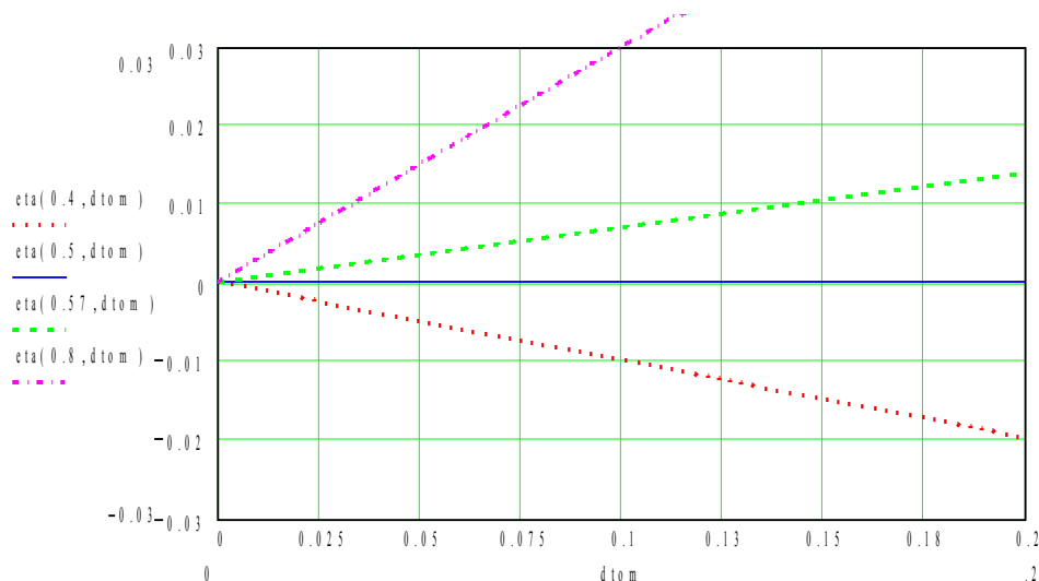
Figure 6.2-a : Coefficient d'amortissement numérique \eta en fonction de \omega \cdot \Delta t \in [0.0, 0.2] , pour \theta = 0.40, 0.50, 0.57, 0.80 .
