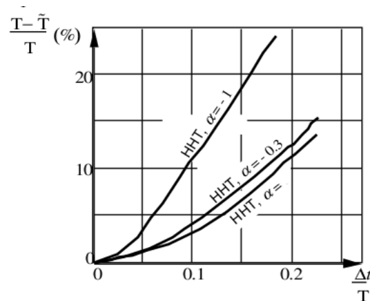
Figure 5.3-b : Erreur relative sur la période en fonction du pas de temps du schéma d'accélération moyenne modifiée
