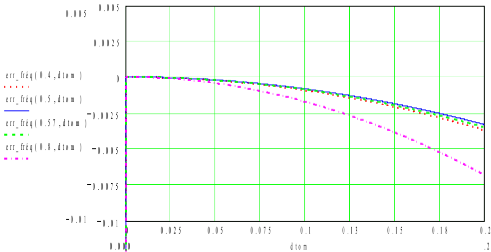
Figure 6.2-c : Erreur en fréquence en fonction de \omega \cdot \Delta t \in [0.0, 0.2] , pour \theta = 0.40, 0.50, 0.57, 0.80 .
