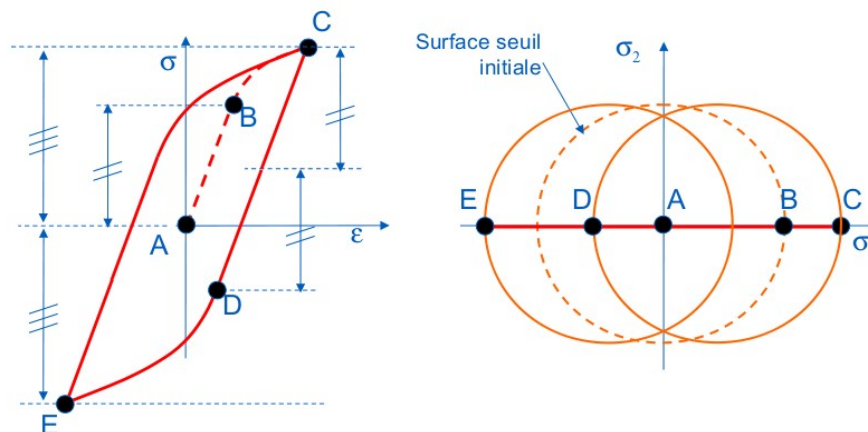
Figure 1.8-2 : Écrouissage cinématique
