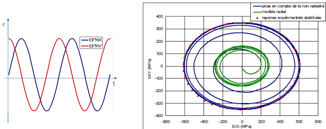
Figure 1.7-1 : Effet de sur-écrouissage sous chargement multiaxial non radial
