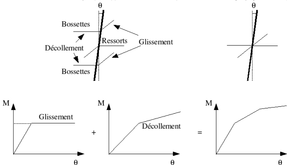
Figüema du comportement de la liaison grille-crayon en rotation.
