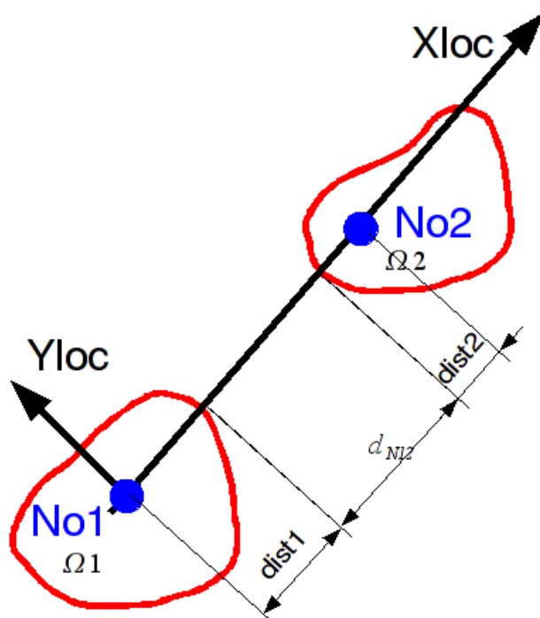
Figure 6.1-a : Définition des distances pour la relation DIS_CHOC.
