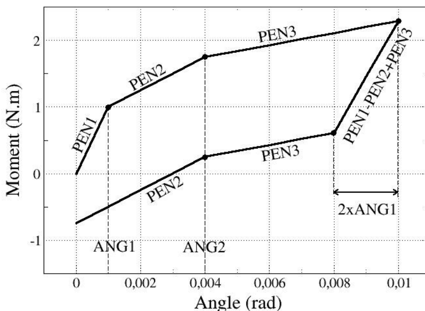
Figure angle-moment sur un essai de charge et décharge en rotation pour la loi DIS_GRICRA.
