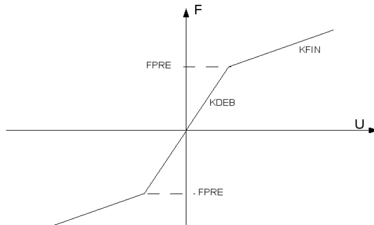
Figure Comportement élastique bilinéaire
