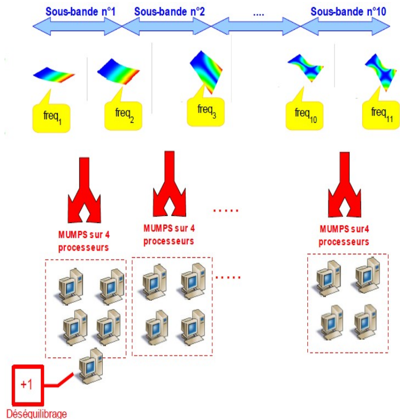
Figure 4-8. Déséquilibre de charge « sous-bandes/processeurs ».
