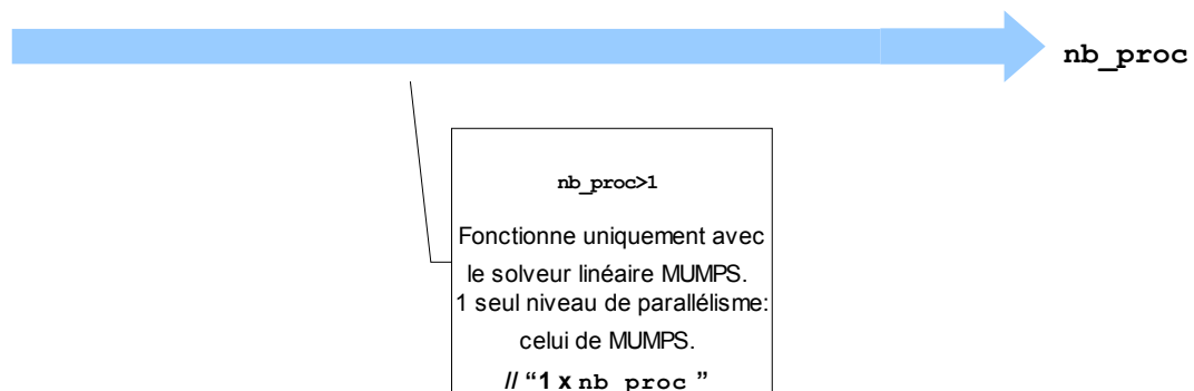
Figure 4-3b. INFO_MODE seul ou en pré-traitement de MACRO_MODE_MECA . Périmètre d'utilisation avec NIVEAU_PARALLELISME ='PARTIEL'.
