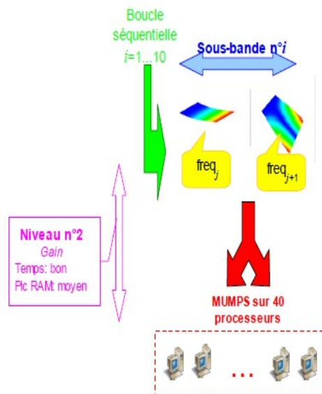
Figure 4-2. Un seul niveau de parallélisme.
