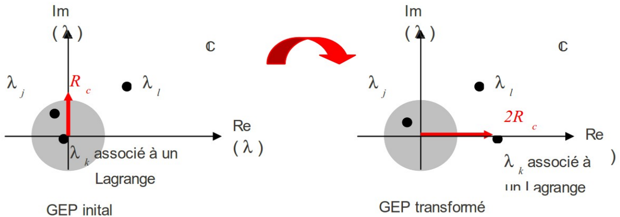
Figure 3.5 Transformation du GEP Aster initial en un GEP compatible avec l'algorithme de Rombouts-Heyde.
