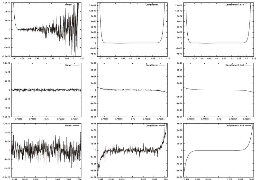
Figure 2.5 Évaluation du polynôme P(\lambda) := (0.75 - \lambda)^5 (1 - \lambda)^{11} dans trois voisinages de ses racines (intervalles [0.68, 1.15] , [0.74995, 0.75005] et [0.9935, 1.0065] ) avec trois méthodes : Horner, Horner compensé et sa version récursive à trois niveaux (extrait de [GLL08]).
