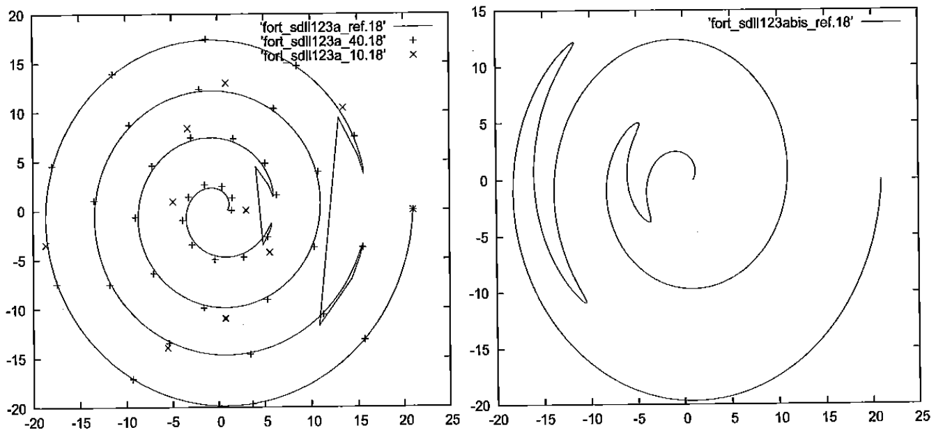
Figure 3.4ab Contours dans le plan P(\lambda) sur le même calcul modal Aster: QEP du cas-test sdll123a.
