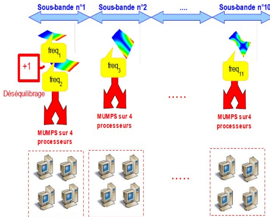
Figure 4-9. Déséquilibre de charge « fréquences/sous-bandes ». INFO_MODE seul ou en pré-traitement de MACRO_MODE_MECA.
