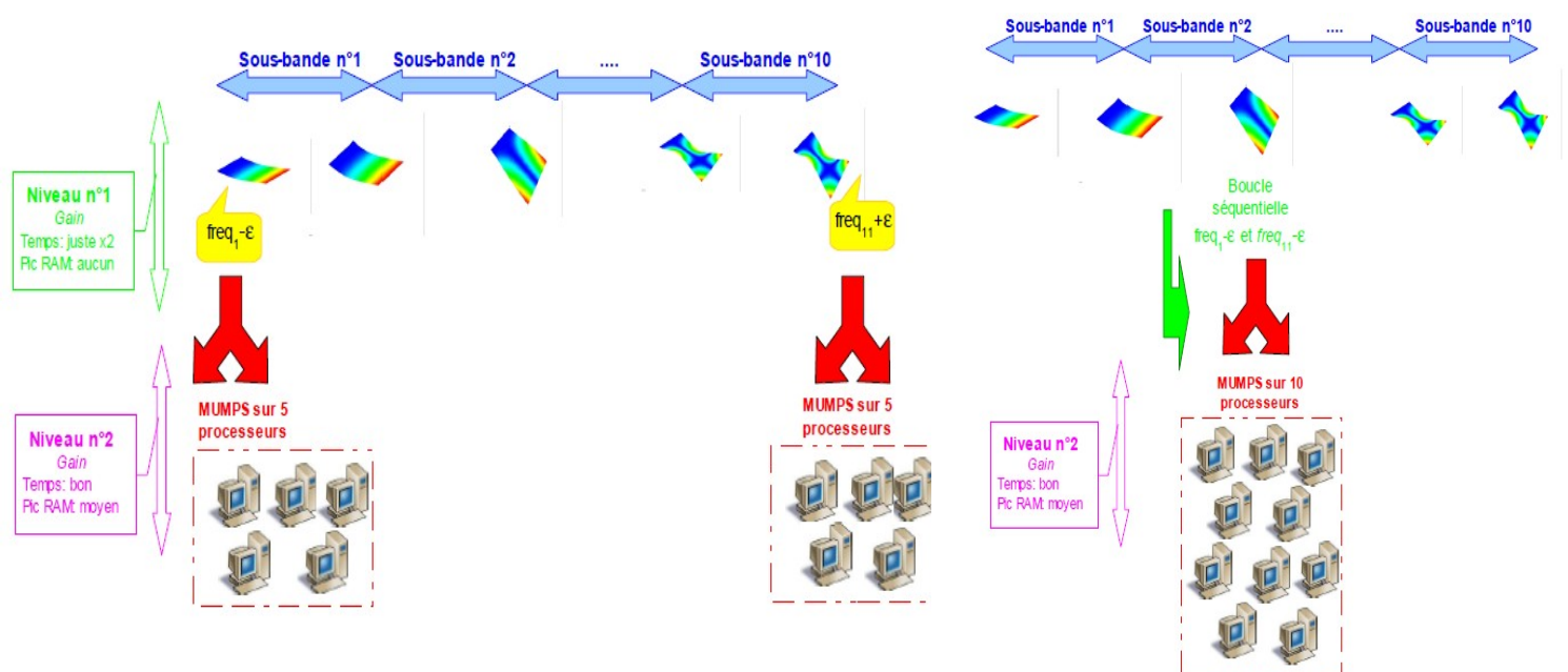
Figure 4-5a/b. Deux ou un seul niveau de parallélisme. INFO_MODE en post-traitement de MACRO_MODE_MECA .
