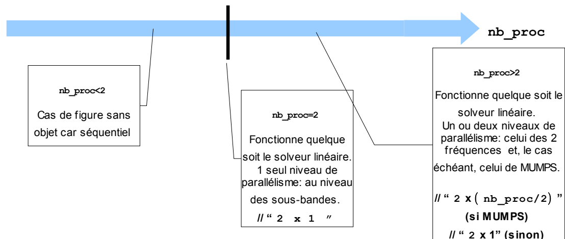
Figure 4-7a. INFO_MODE de post-traitement de MACRO_MODE_MECA . Périmètre d'utilisation avec NIVEAU_PARALLELISME ='COMPLET'.
