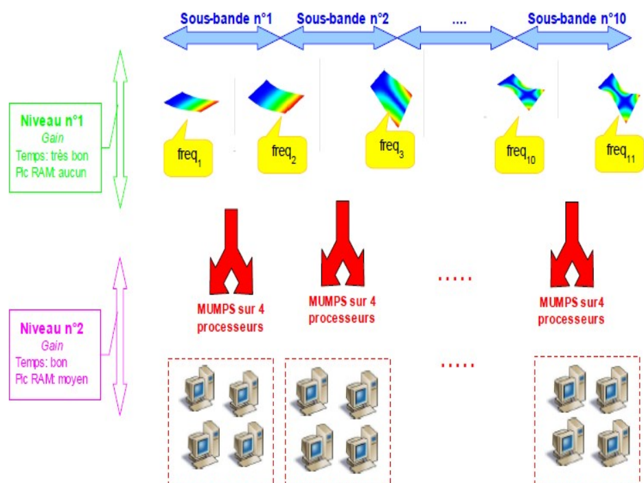
Figure 4-1. Deux niveaux de parallélisme.
