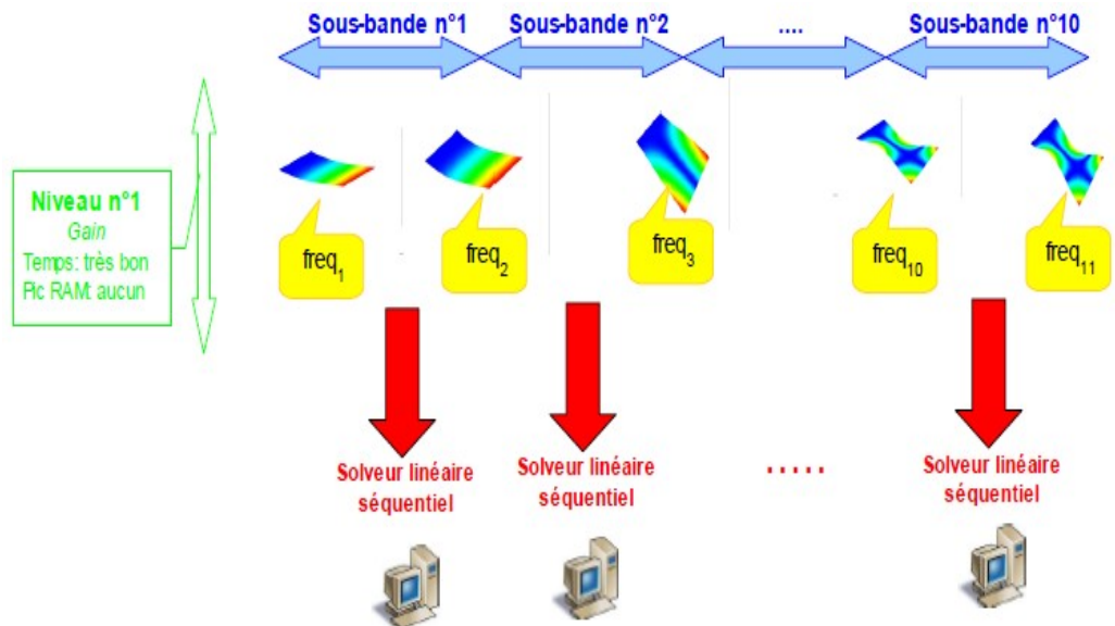
Figure 4-4. Un seul niveau de parallélisme.
