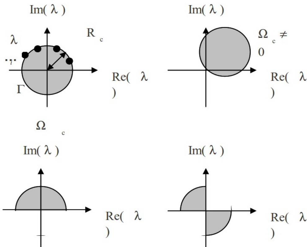
Figure 3.1abcd Différentes formes de domaine de contrôle pour la méthode APM.
