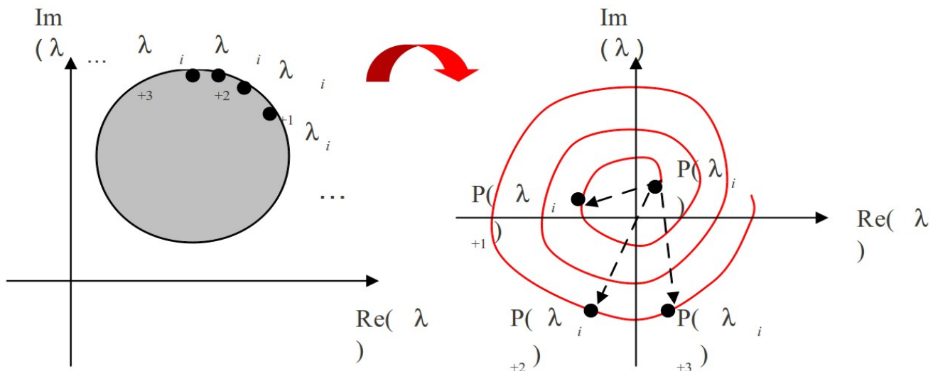
Figure 3.3 Problématique de la discrétisation du contour afin de capter tous les tours de la courbe fermée. Ici l'arc de cercle \lambda_{i+1} \lambda_{i+2} n'est pas assez discrétisé, on rate un tour ! Donc la vérification sera faussée.
