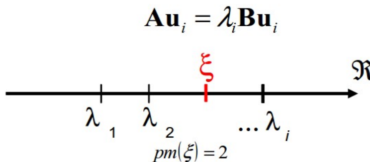
Figure 2.1 Test de Sturm de Code_Aster : principe des suites de Sturm appliqué au GEP standard.
