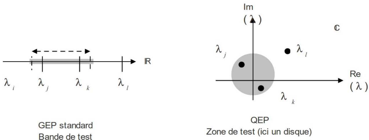
Figure 1.1 Deux problématiques distinctes: dénombrement des valeurs propres contenues strictement dans un segment de l'axe réel et dans une portion finie du plan complexe.
