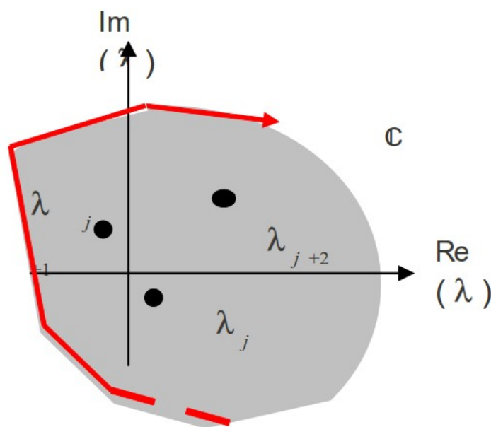
Figure 3.2 Méthode de continuation pour construire, « en temps réel », le domaine « optimisé » (contrôle a posteriori).
