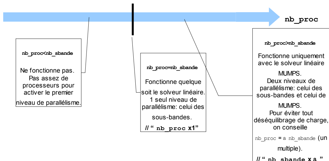
Figure 4-3a. INFO_MODE seul ou en pré-traitement de MACRO_MODE_MECA . Périmètre d'utilisation avec NIVEAU_PARALLELISME='COMPLET' .
