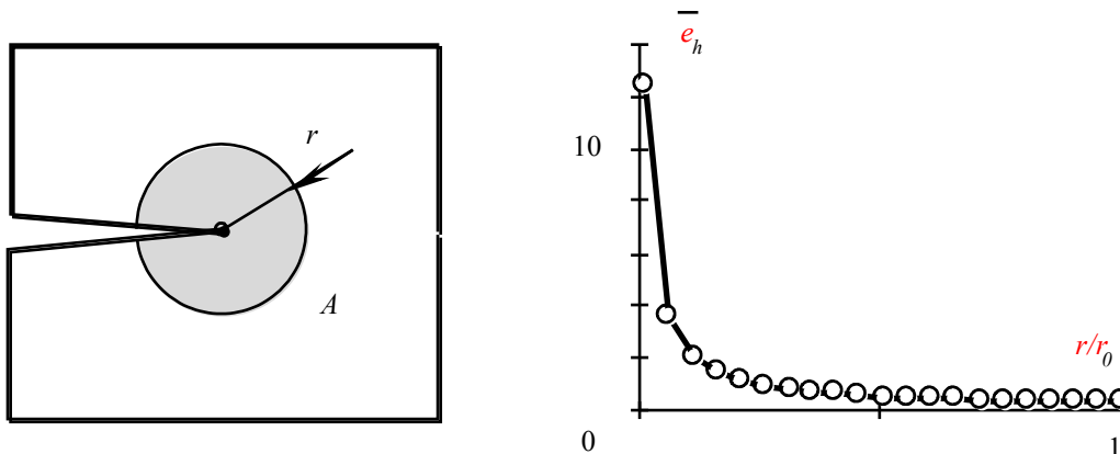
Figure 2.3.1-a : Evaluation numérique de \alpha
