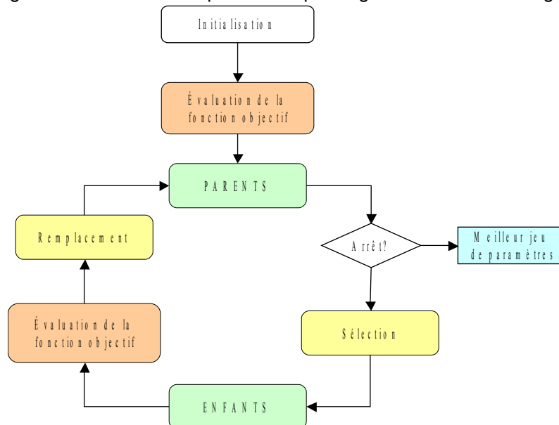
Figure 3.2-a Schéma logique du fonctionnement de l'algorithme évolutionnaire
