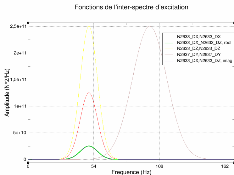
Figure 5.2.1-a : inter-spectre d'excitation.
