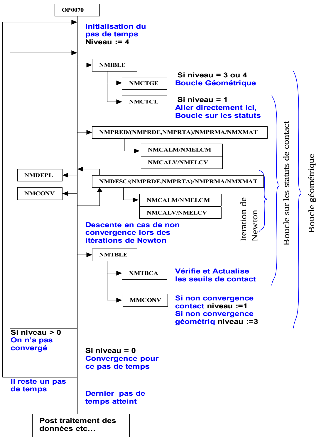
Figure 5. L'arbre d'appel de l'opérateur STAT_NON_LINE pour le traitement d'un problème de contact en grands glissements avec XFEM.
