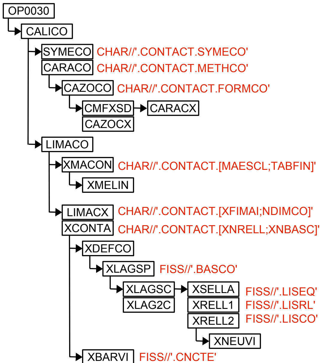
Figure 3. L'arbre d'appel de l'opérateur DEFI_CONTACT pour le mot clé FORMULATION='XFEM'
