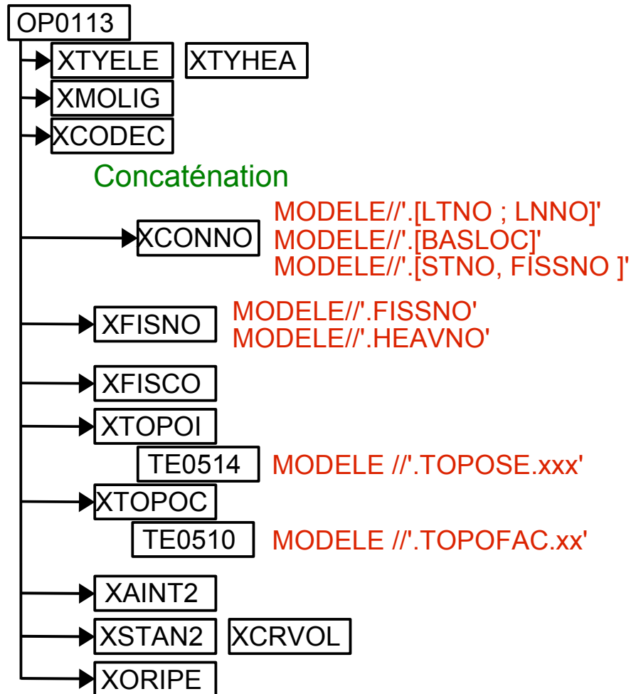
Figure 2. L'arbre d'appel de l'opérateur MODI_MODELE_XFEM
